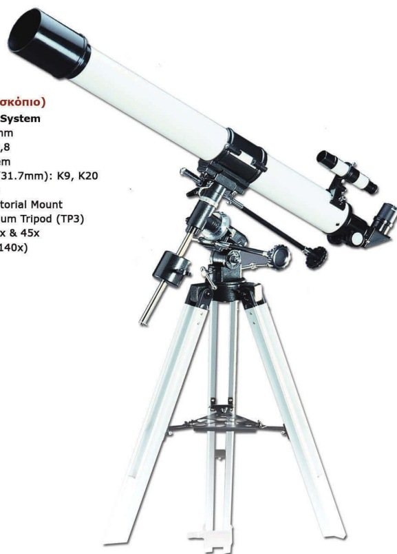
120206 (Κατοπτρικό-Νευτώνειο Τηλεσκόπιο) Telescope Newton - Spherical Reflector System F= 1000mm D=114mm Focus Ration: F 8,8 Eyepieces (1.25"/31.7mm): K9, K20 Finderscope: Red Dot Βάση: EM9 Equatorial Mount Τρίποδα: Aluminum Tripod (TP3) Μεγένθυση: 111x & 50x (Μέγιστη ιδανική:222x) EXTRA:
